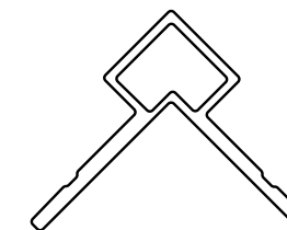
Bordure de coin extérieur UH60 127 x 127 mm (5 x 5 po)
